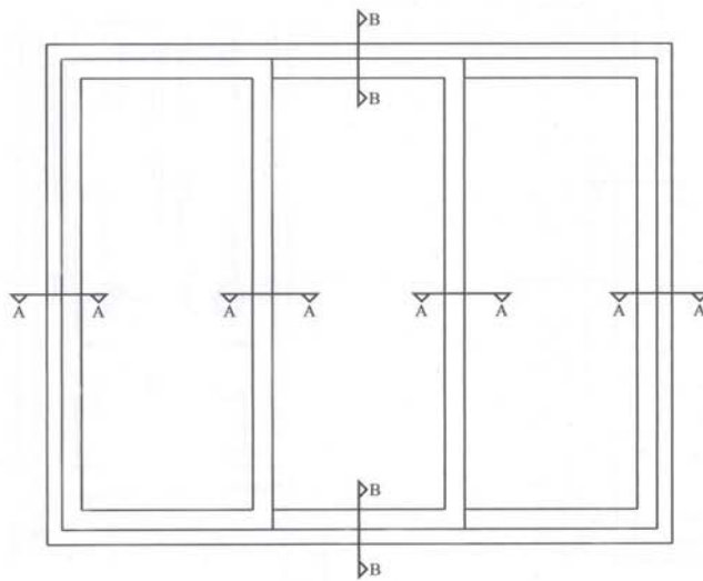
ELEVATION
